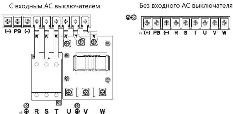
Рис 4.10 Силовые клеммы 18 – 22 кВт (G-тип)
