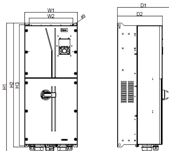
Рис С.2 Схема настенного монтажа ПЧ моделей 45-110 кВт (G-тип)
