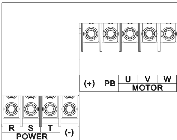
Рис 4.13 Силовые клеммы 75 – 110 кВт (G-тип)
