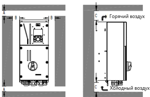
Рис 4.3 Одиночная установка
