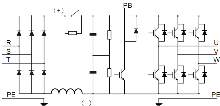
Рис 3.2 Схема силовой цепи моделей 18-110 кВт (G-тип)
