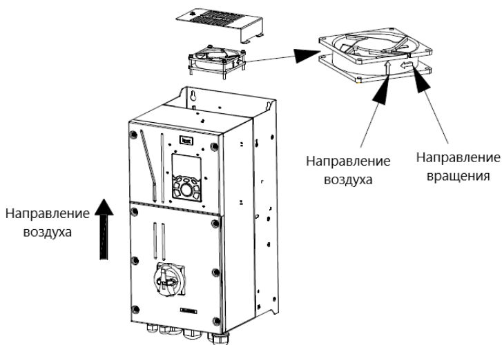
Рис 8.1 Обслуживание вентиляторов для инверторов мощностью 7,5 кВт или выше (G-тип)
