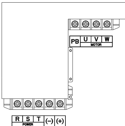
Рис 4.12 Силовые клеммы 45 – 55 кВт (G-тип)
