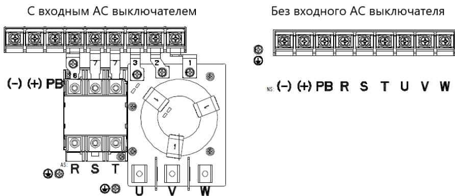
Рис 4.11 Силовые клеммы 30 -37 кВт (G-тип)
