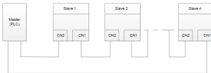
Рисунок А.10 Электрическая схема подключения кольцевой сети
