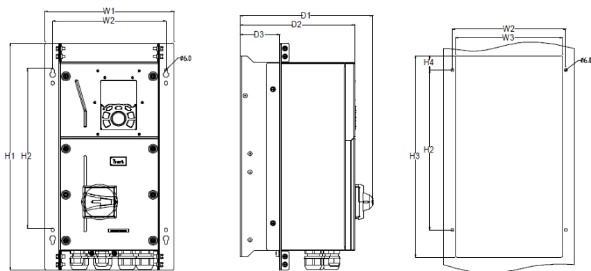
Рис С.3 Схема фланцевого монтажа ПЧ моделей 4-37 кВт (G-тип)
