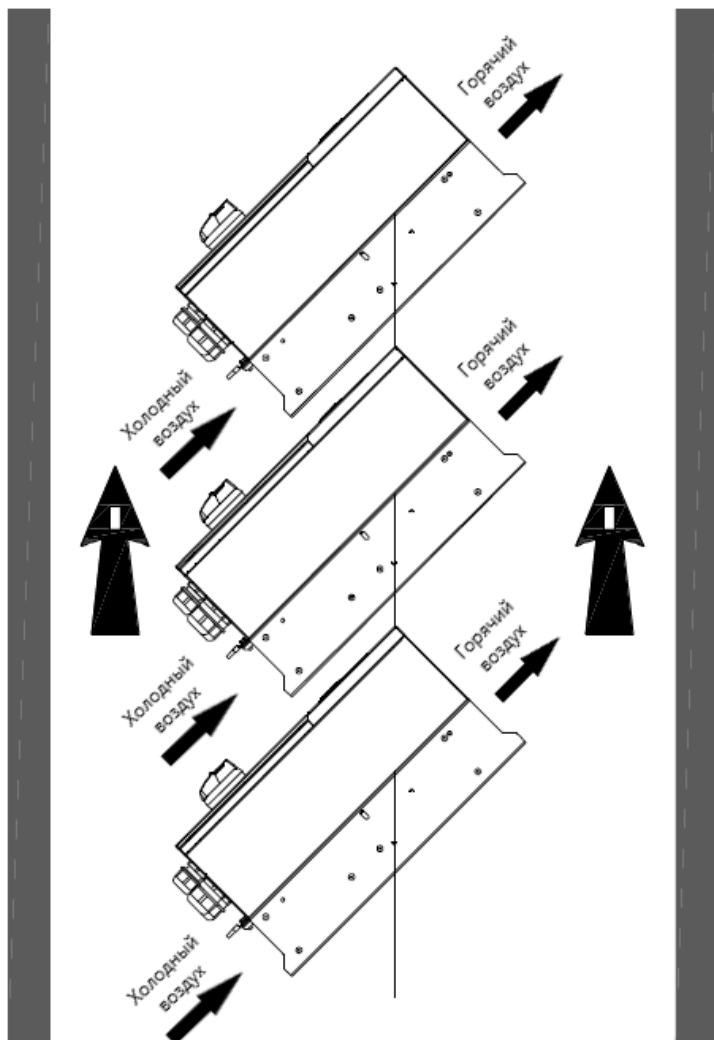
Рис 4.6 Наклонная установка
