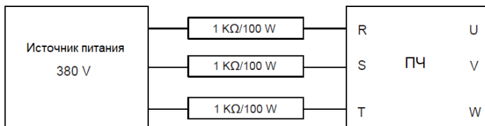
Рисунок 8.1 Пример схемы зарядки ПЧ
