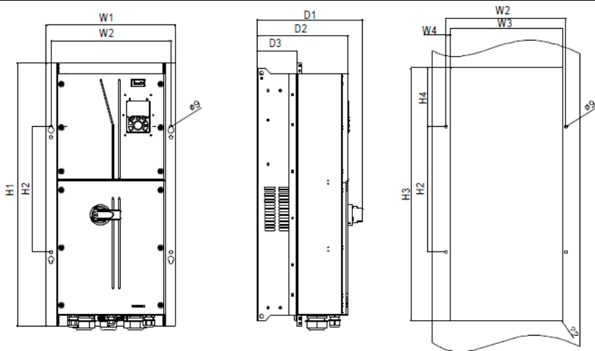
Рис С.4 Схема фланцевого монтажа ПЧ моделей 45-55 кВт (G-тип)
