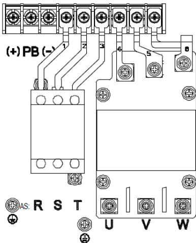
Рис 4.8 Силовые клеммы 4 – 5,5 кВт (G-тип)
