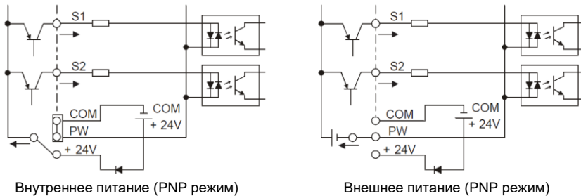
Рис 4.18 PNP режим
