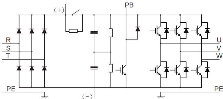
Рис 3.1 Схема силовой цепи моделей 15 кВт и ниже (G-тип)
