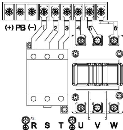
Рис 4.9 Силовые клеммы 7,5 – 15 кВт (G-тип)
