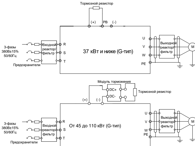
Рис 4.7 Схема подключения силовой цепи
